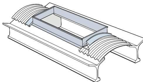
INSTALLAZIONI SU COPERTURA CON TRAVE A "Y"
